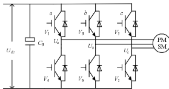
图 2-8 逆变电路
